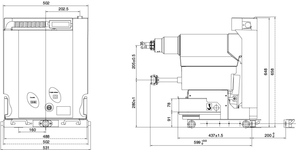
固定式真空接触器
